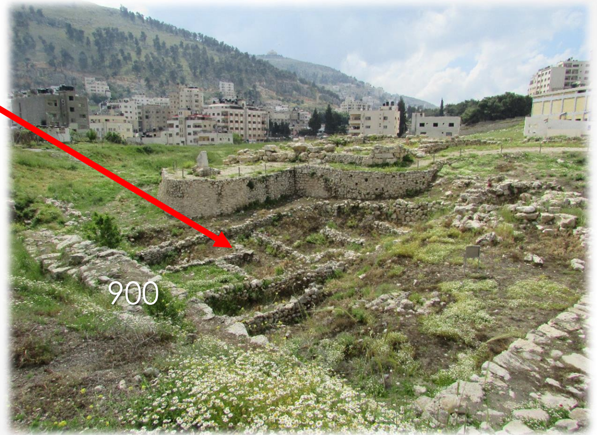
Die Mauer 900 und die Tempelanlage aus der MBIIA (2000 – 1750 v. Chr.)
